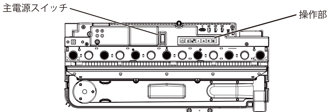
CAS500P-RGB-J 内部ユニット上面
