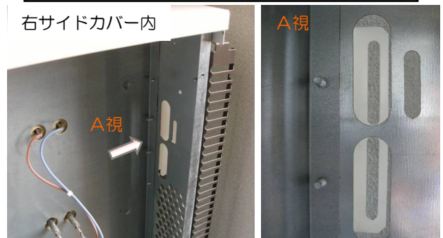
③壁固定金具-壁固定方法（正面視右側1箇所）
