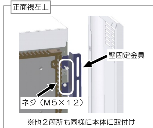
①壁固定金具-本体取付け方法（背面視）
