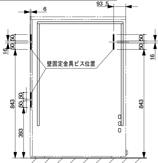
②壁固定金具-壁固定方法（正面視左側2箇所）
